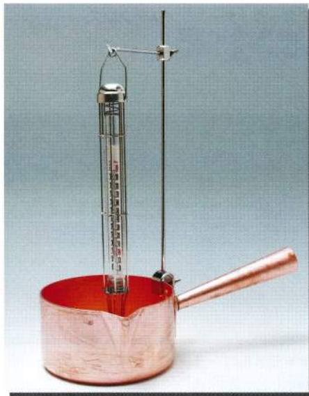
温度計ハンガー 130590 320 ガード付き温度計 130571 80~200℃
