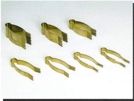
マジバンつまみ 洋銀 278007 L55×W4~25 7本セット
