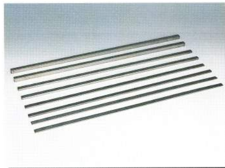
パール(8本セット) ステンレス 310252 2×10×500、3×10×500 5×10×500、10×10×500 各2本
