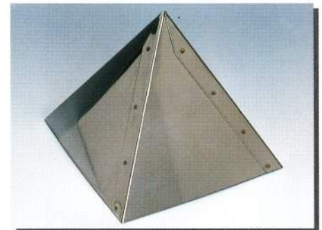
ピラミッド ステンレス 72571 L40 × 40 H35 18cc 72572 50 × 50 43 38 72573 60 × 60 52 62 72575 120 × 120 104 490 72576 140 × 140 120 790 72577 160 × 160 138 1200
