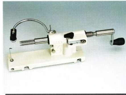
皮むき器 102200 340×190×70 皮むき・スライス・芯を取り除く
