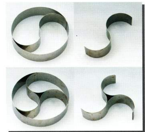
マガタマ 2ヶ取り マガタマ 3ヶ取り 315402 φ150×40H 315403 φ150×40H 315452 150×45 315453 150×45 318402 180×40 318403 180×40 318452 180×45 318453 180×45 321402 210×40 321403 210×40 321452 210×45 321453 210×45
