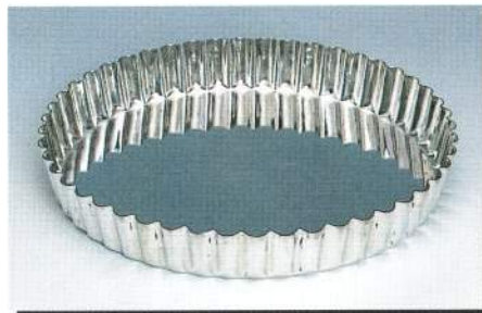
タルト スズメッキ フッ素樹脂加工 73230 673230 φ 140/130 H20 73231 673231 160/150 20 73233 673233 180/170 25 73235 673235 200/190 25 73237 673237 220/210 25 73239 673239 240/230 25 73241 673241 260/250 25 73243 673243 280/270 25 73245 673245 300/290 25 73247 673247 320/310 25
